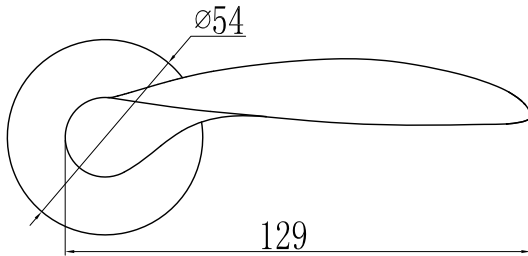
SOLID – HS3062-EN4L
